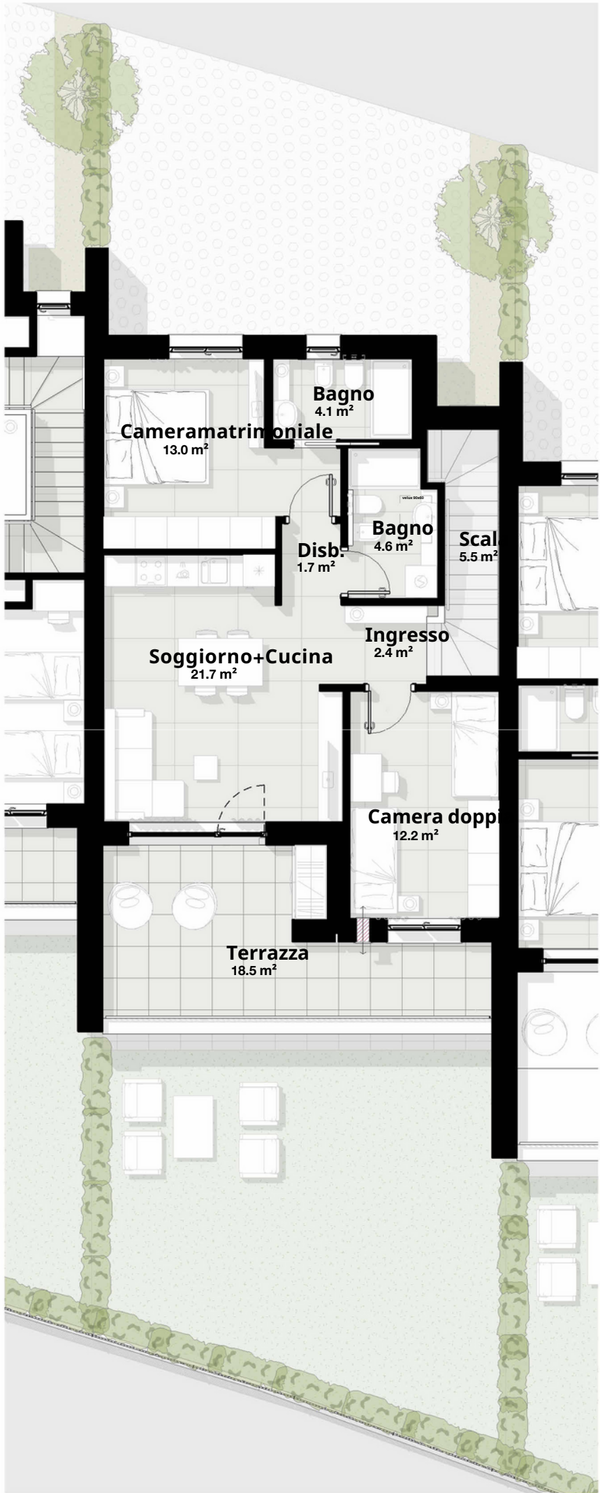
PIANO PRIMO Pianta 1:100
